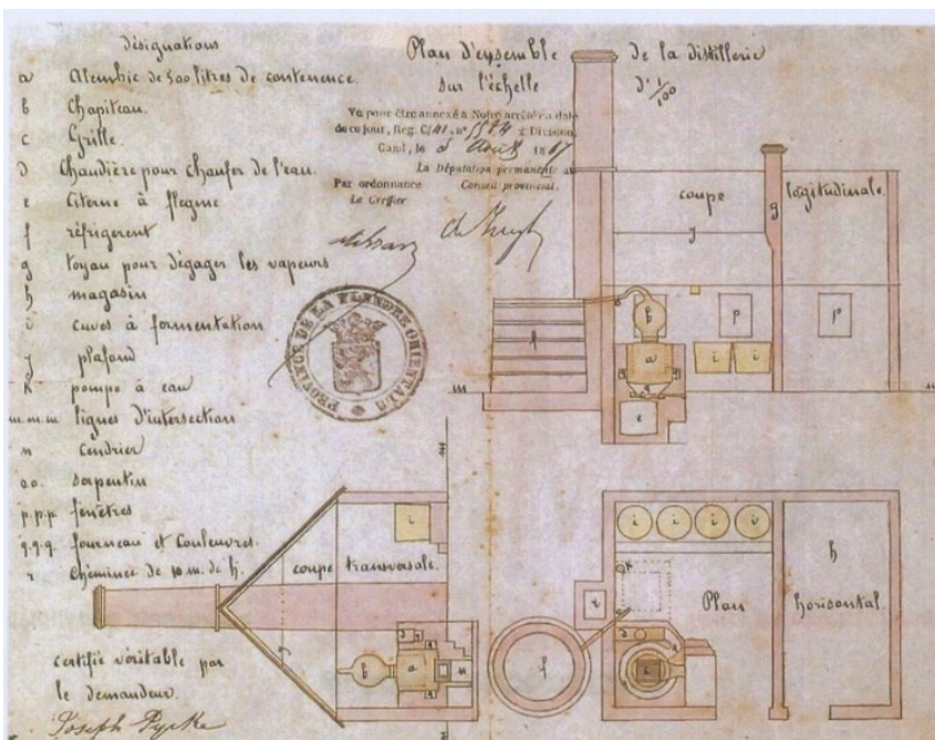
Grondplan ((1867) van de landbouwtokerij Pycke uit Sint Kornelis-Horebeke met bovenaanzicht, zijzicht en dwarsdoornede. Tijdens de 18de eeuw waren de meeste landbouwtokerijen op deze wijze ingericht. Figuur uit de privécollectie van Prof. Dr. Eric Van Schoonenbergh
