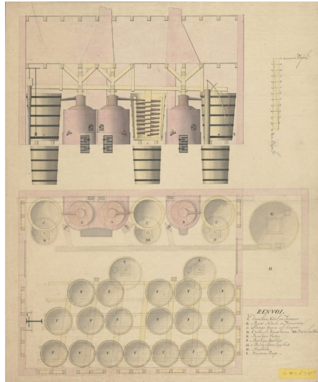
Grondplan & doorsnede van de branderij “Hollandse wijze” De Papegaay in Delft. Dergelijke stokerijen werden ook in de Zuidelijke Nederlanden opgericht.
